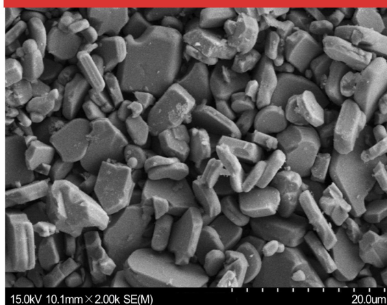
电镜图 SEM
