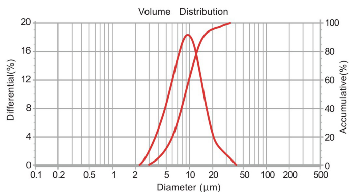
粒径分布 Particle Size Distribution
