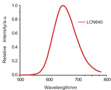
发射光谱 EM Spectrum
